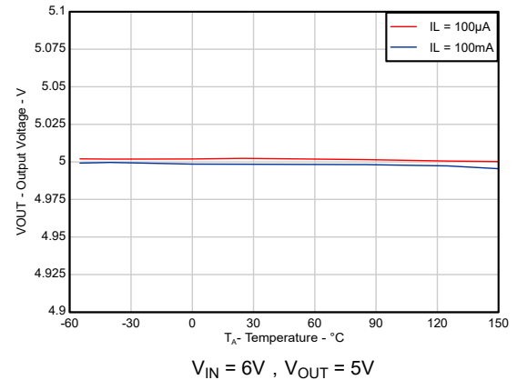
图 5-10. 输出电压与温度之间的关系 (新芯片)
