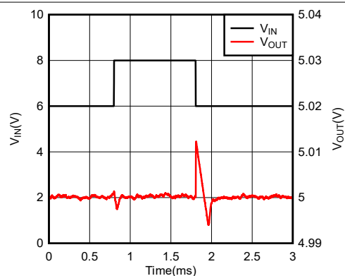
图 7-6. 线路瞬态响应与时间之间的关系 (新芯片)
