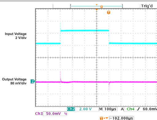
图 7-5. 线路瞬态响应与时间之间的关系 (旧芯片)
